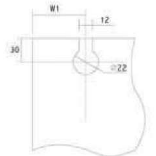
► KZNİ-8600C-1 SÜRME KAPI TEKERLEĞİ Cam Delik Ölçüleri
